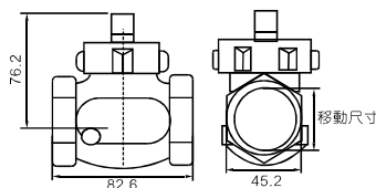
尺寸 (mm)
