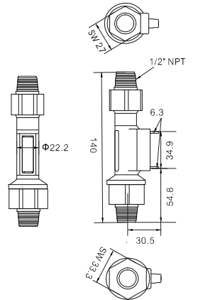
尺寸 (mm)
