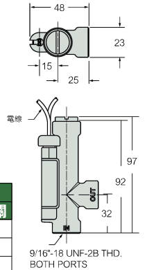
尺寸 (mm)
